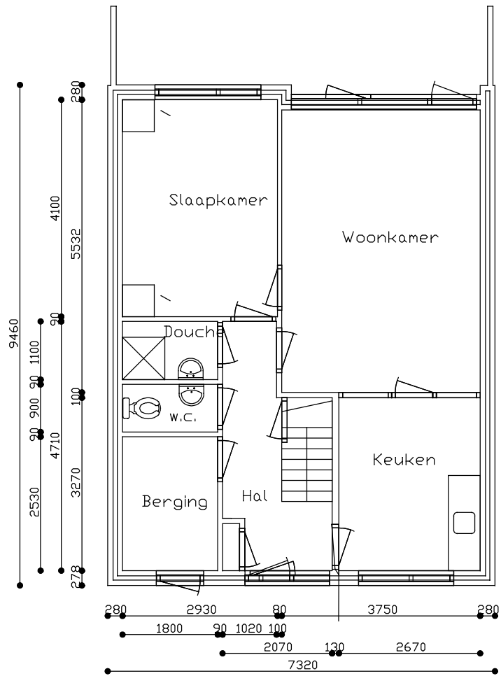
Begane grond
