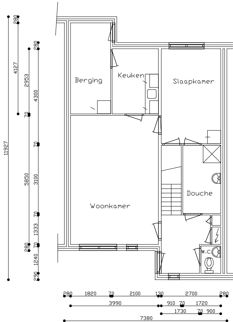
Begane grond
