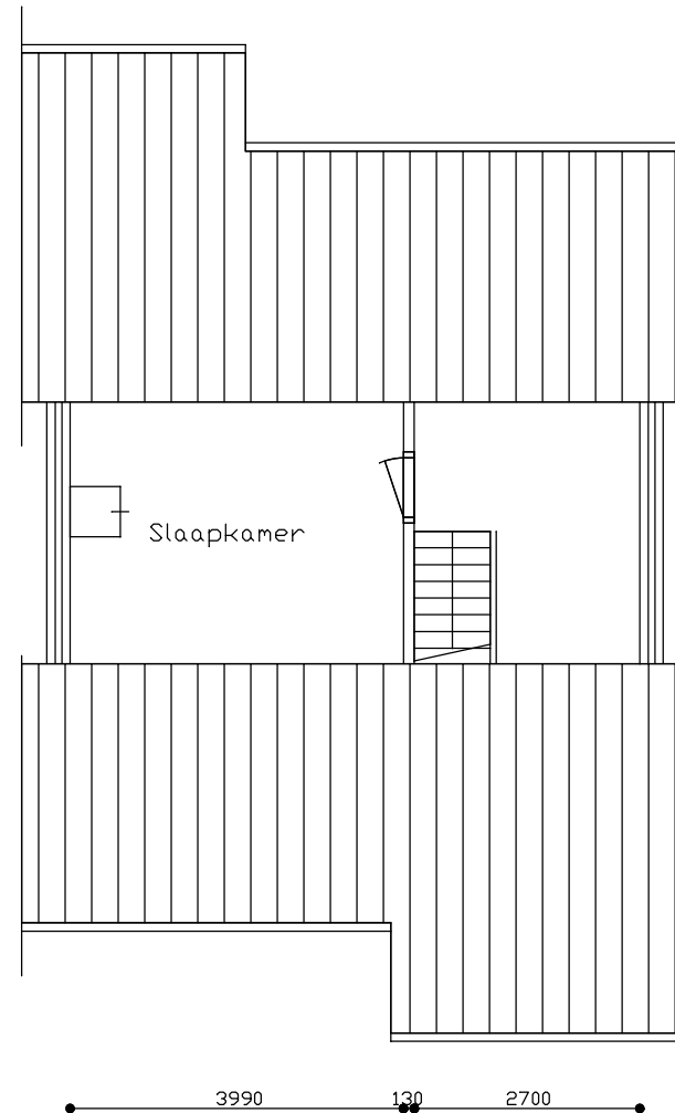
Verdieping
